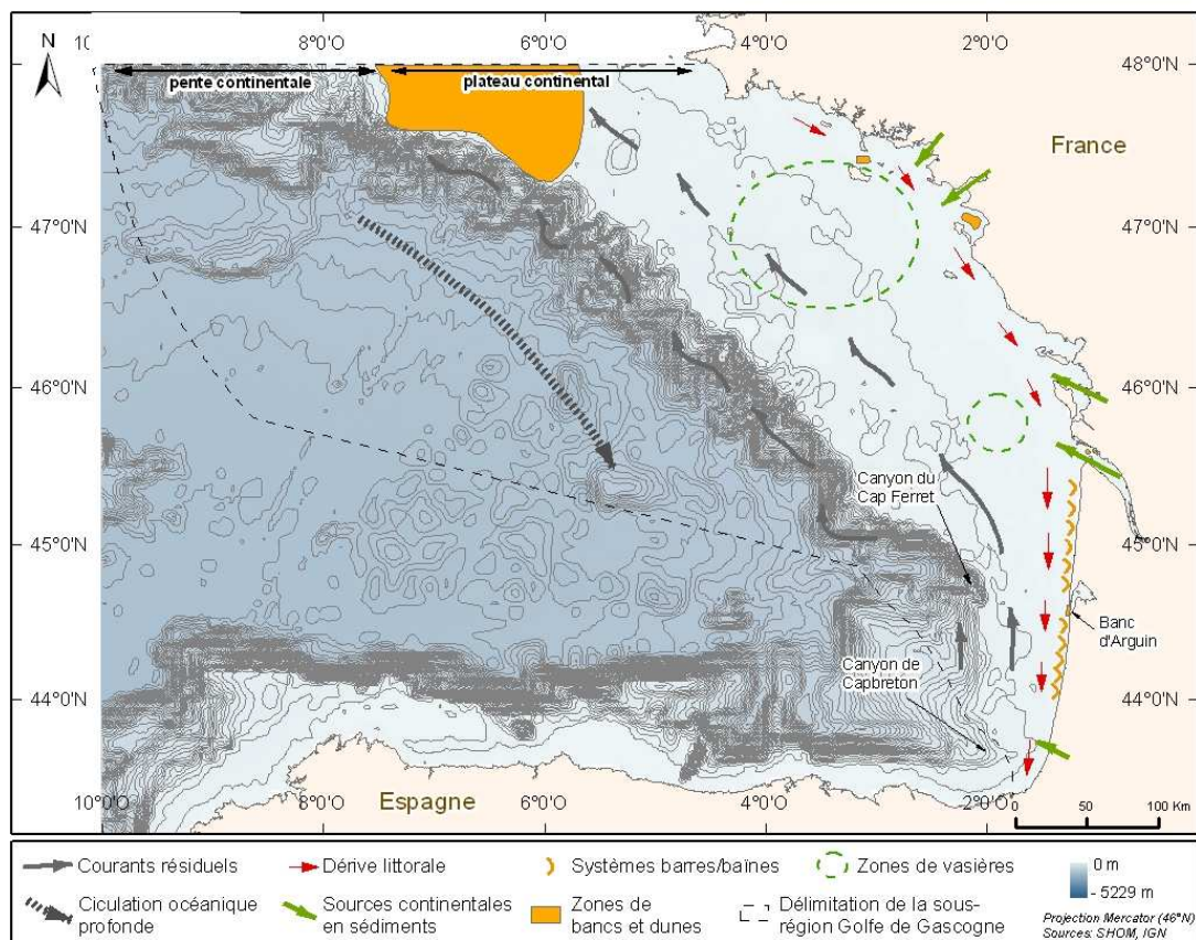
Figure 1 : Principaux transits sédimentaires et localisation des principales structures du Golfe de Gascogne
